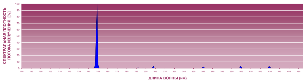
Безозоная бактерицидная лампа Относительное спектральное распределение энергии
